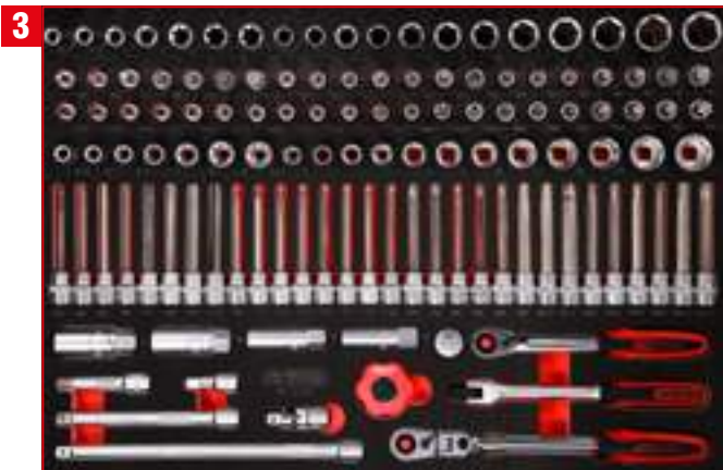
3/8" Steckschlüssel-Satz
